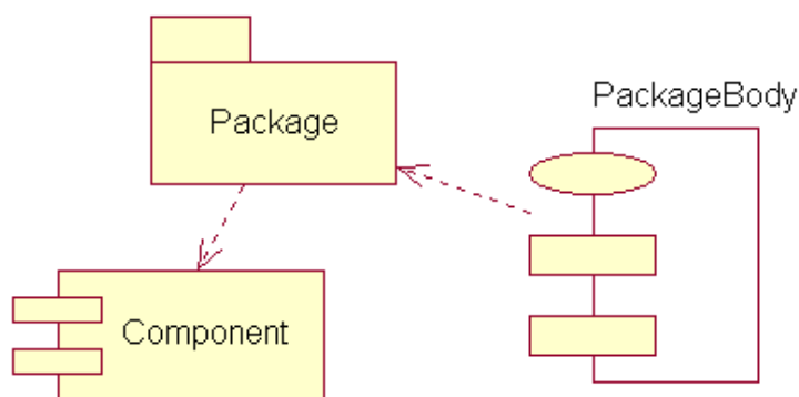
Рис.8. Диаграмма классов
