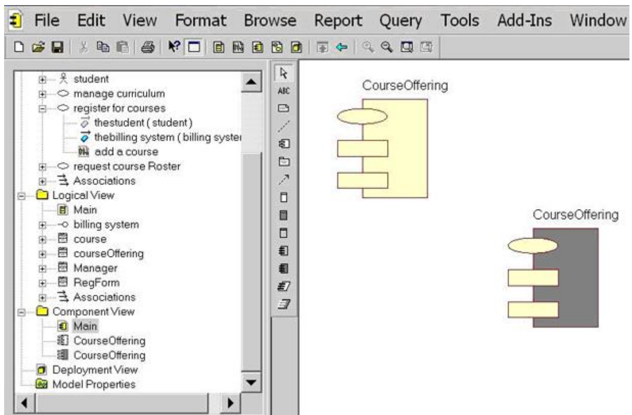
Рис. 22. Диаграмма компонентов
