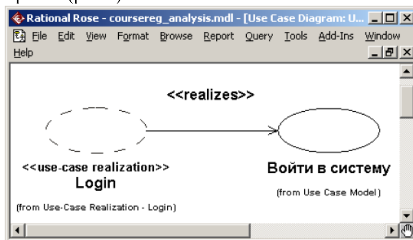
Рис.4. Диаграмма трассировки
