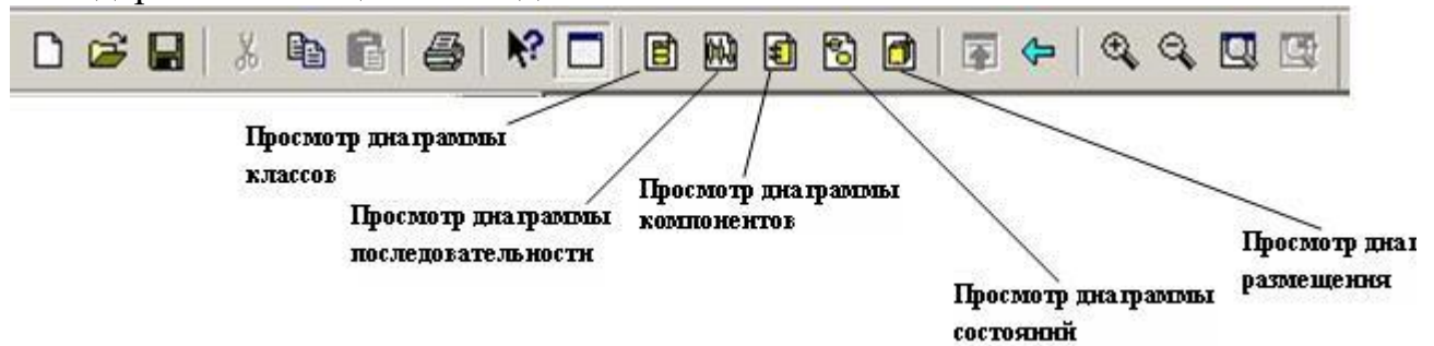
Рис. 3. Строка инструментов.
